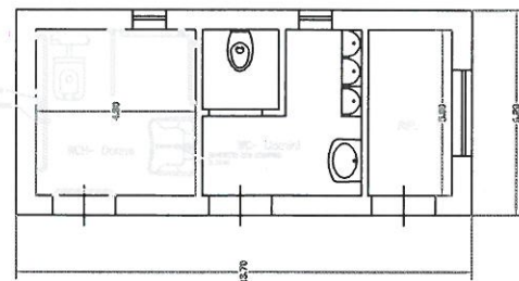
Pianta servizi igienici
